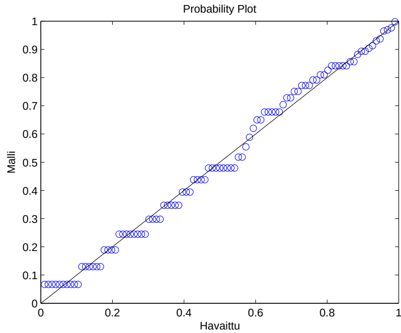
Kuva 2.25: Todennäköisyyskuvaaja tason u = 96 cm ylitteiden GPD-sovitteelle.
