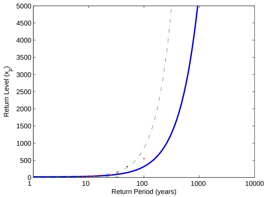
Kuva 3.34: Onnettomuuskuolemien toistumistasokuvaaja GPD-mallissa ( u = 30 ) luottamusväleihin; yhdistetty aineisto.
