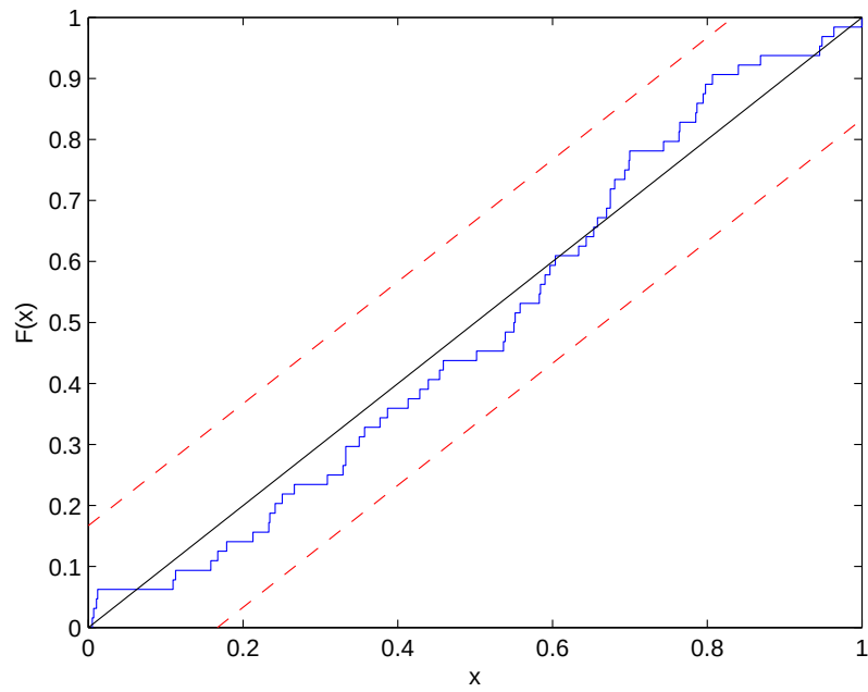
Kuva 3.12: Muunnettuihin odotusaikoihin perustuvan suureen U_k empirinen jakauma (sininen viiva) tasajakaumaa vastaan luottamusväleinen; u = 3 .
