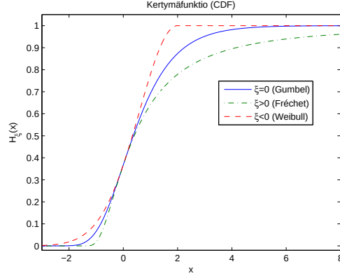
Kuva 1.2: GEV-jakauman kertymäfunktio.
