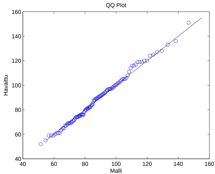
Kuva 2.8: Kvantiilikuvaaja vuosimaksimien GEV-sovitteelle.
