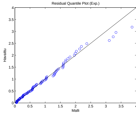
Kuva 2.51: Kvantiilikuvaaja mallille \mathcal{M}_2 .
