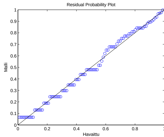
Kuva 2.40: Todennäköisyyskuvaaja POT-mallille ( u = 96 ).
