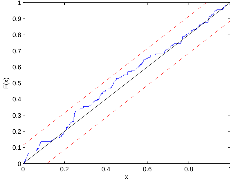
Kuva 3.28: Muunnettuihin odotusaikoihin perustuvan suureen U_k empirinen jakauma (sininen viiva) tasajakaumaa vastaan luottamusväleinen; u = 3 .
