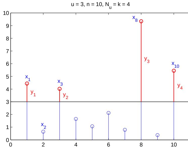
Kuva 2.16: Ylitteen menetelmän datan havainnollistus: havaittu otos \mathbf{X} = \mathbf{x} ja tason u = 3 ylitteet \mathbf{Y} = \mathbf{y}
