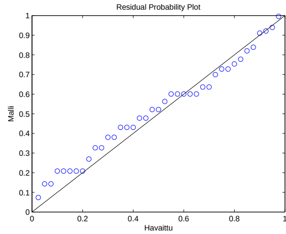
Kuva 2.42: Todennäköisyyskuvaaja POT-mallille ( u = 108 ).
