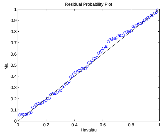
Kuva 2.56: Todennäköisyyskuvaaja mallille \mathcal{M}_2^N .
