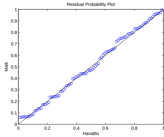
Kuva 2.48: Todennäköisyyskuvaaja mallille \mathcal{M}_1 .
