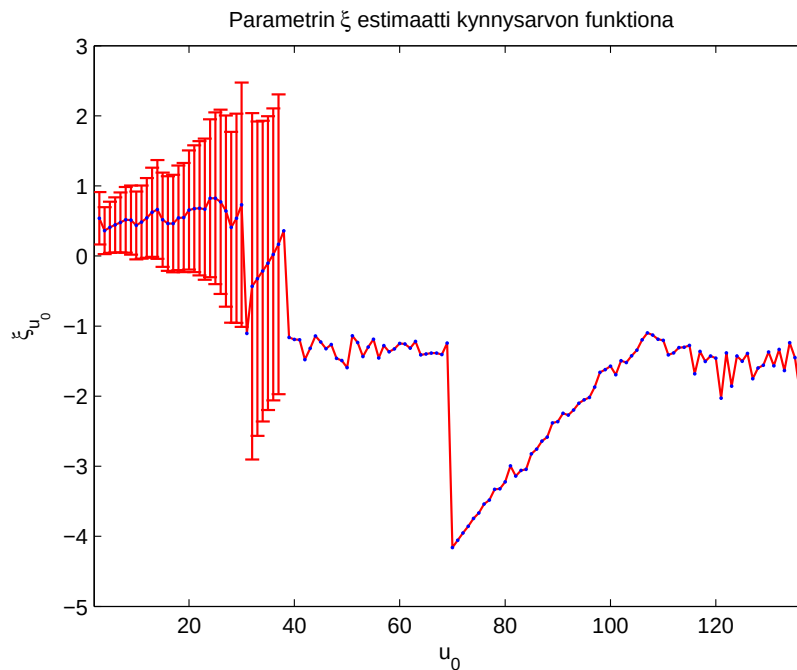
Kuva 3.7: Parametrin \xi estimaatti onnettomuuskuolemadataan sovitetulle GP-jakaumalle kynnyksarvon funktiona.
