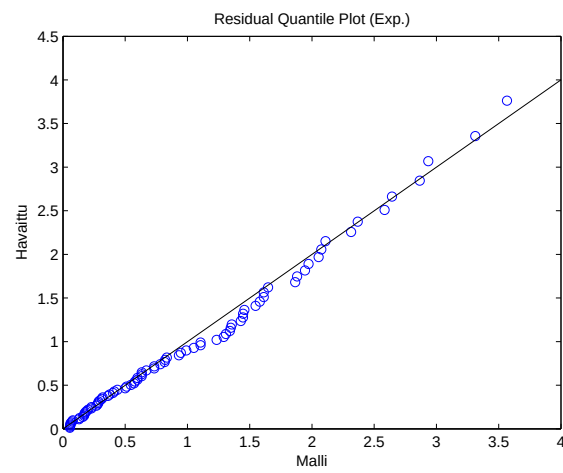
Kuva 2.57: Kvantiilikuvaaja mallille \mathcal{M}_2^N .
