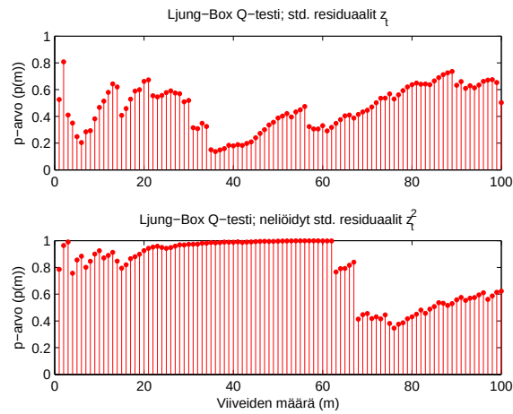
Kuva 4.4: Ljung-Box-testin p -arvot eri viivemäärillä m .
