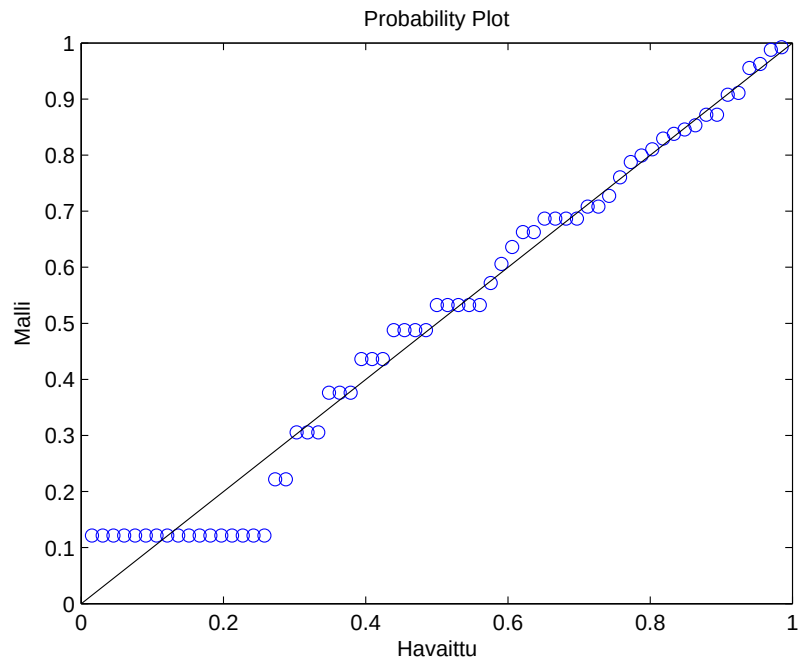
Kuva 3.19: Todennäköisyyskuvaaja onnettomuuskuolemadataan sovitetulle GP-mallille; u = 3 .
