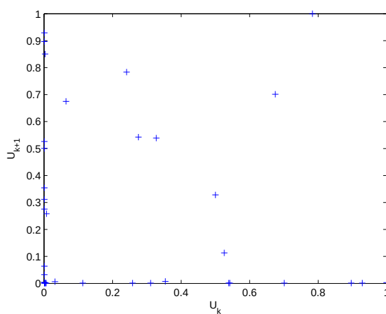
Kuva 2.47: U_k vs. U_{k+1} ; u = 108 .
