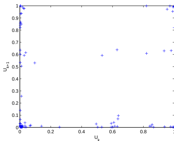
Kuva 2.46: U_k vs. U_{k+1} ; u = 96 .
