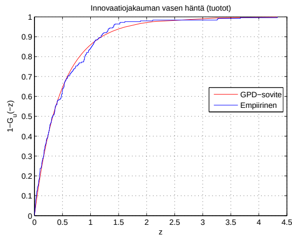
Kuva 4.8: Innovaatiojakauman vasen häntä, vastaten voittoja.
