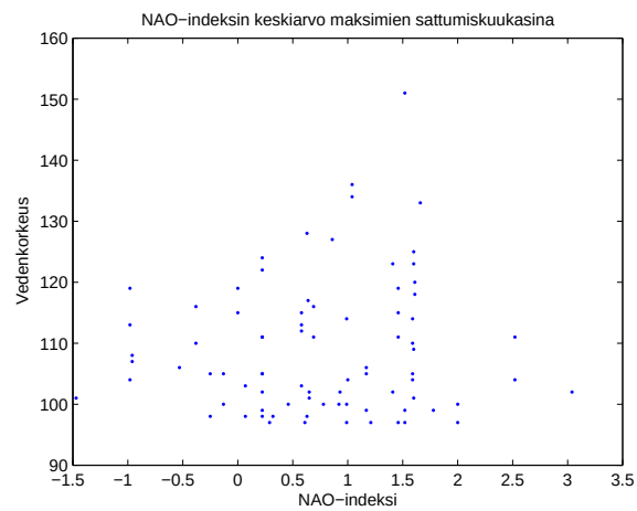
Kuva 2.53: Tason u = 96 cm ylittävät vedenkorkeushavainnot piirrettynä sattumiskuukauden NAO-indeksin keskiarvoa vasten.
