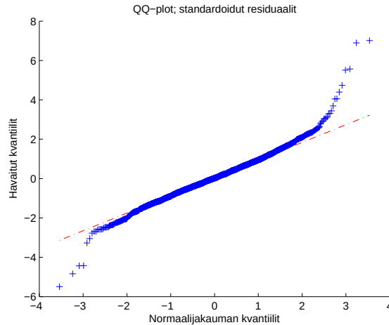
Kuva 4.5: Kvantiilikuvaaaja; standardoidut residuaalit vs. normaalijakauma.
