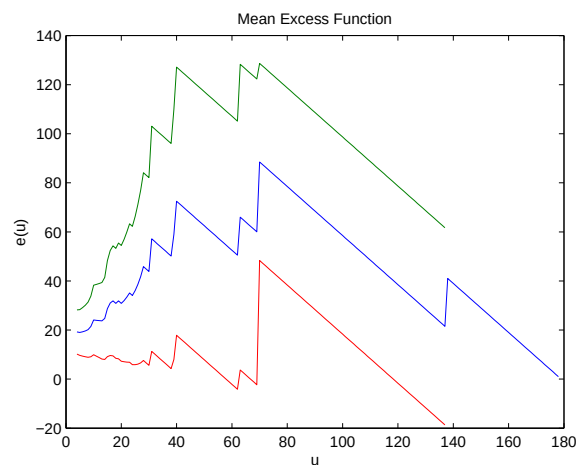
Kuva 3.6: Ylitteen otoskeskiarvokuvaaja onnettomuuskuolematilalle.
