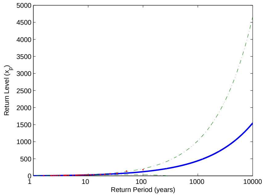
Kuva 3.22: Onnettomuuskuolemien toistumistasokuvaaja GPD-mallissa ( u = 3 ) luottamusväleinen.
