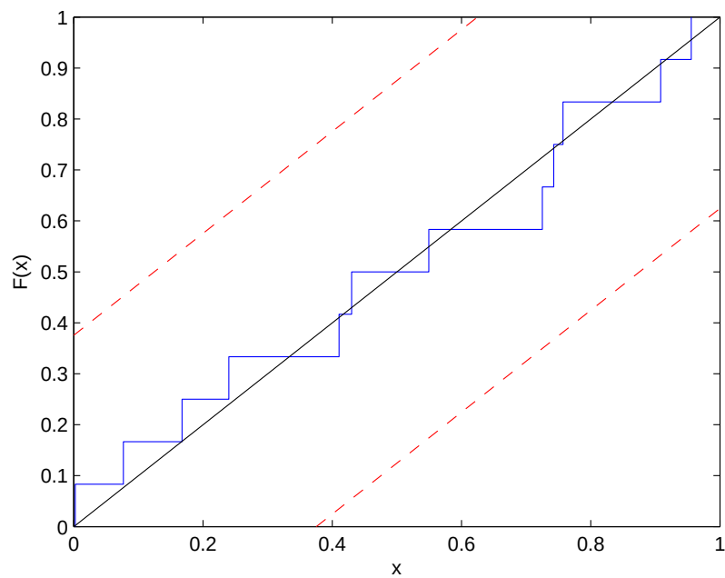
Kuva 3.27: Muunnettuihin odotusaikoihin perustuvan suureen U_k empiirinen jakauma (sininen viiva) tasajakaumaa vastaan luottamusväleinen; u = 30 .
