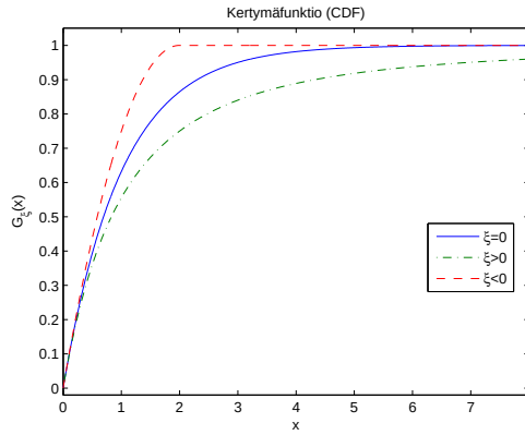
Kuva 1.4: GP-jakauman kertymäfunktio.
