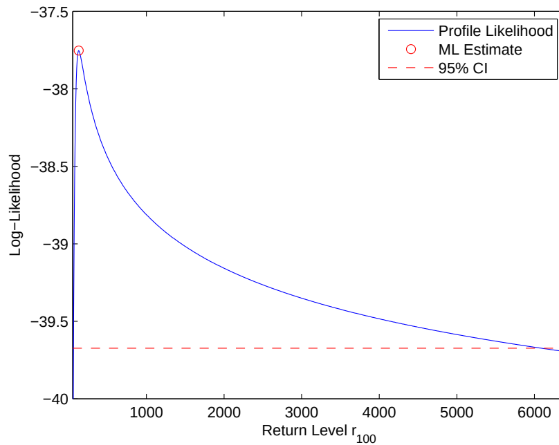
Kuva 3.35: Profiiliuskottavuus onnettomuuskuolemien 100-vuoden toistumistasolle yhdistettyyn aineistoon perustuvassa GPD-mallissa ( u = 30 ).
