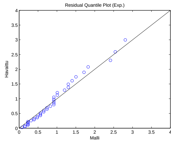
Kuva 2.43: Kvantiilikuvaaja POT-mallille ( u = 108 ).
