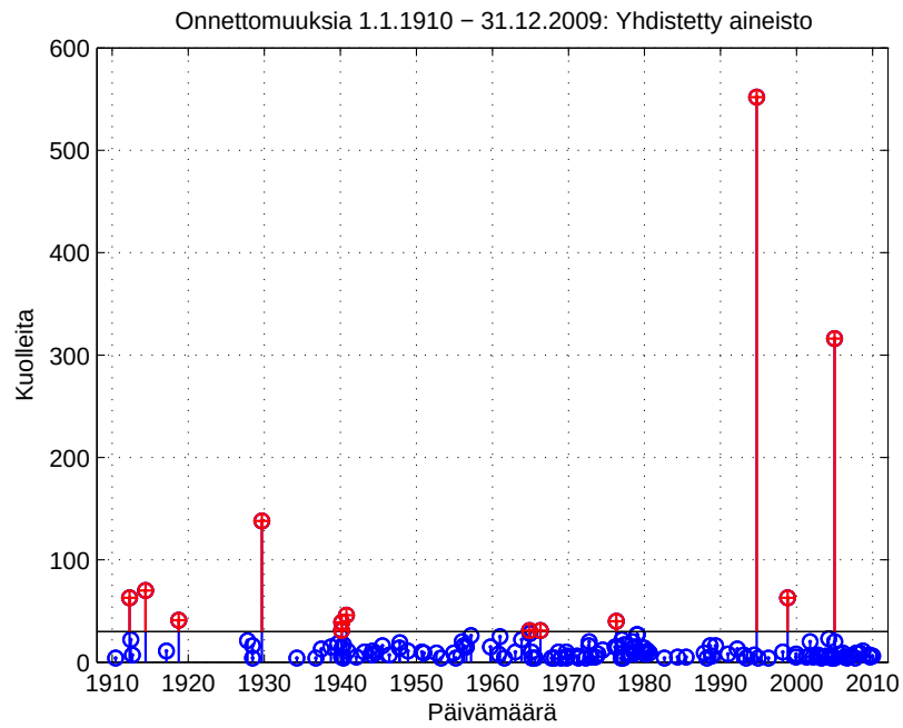
Kuva 3.26: Yhdistetty onnettomuuskoulemadata ja tason u = 30 ylitteet.
