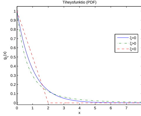
Kuva 1.3: GP-jakauman tiheysfunktio.
