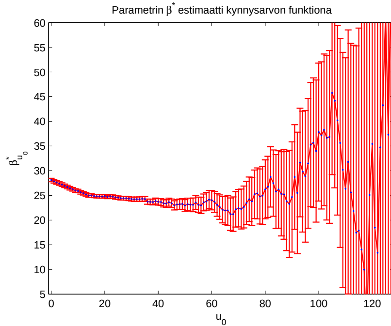
Kuva 2.20: Parametrin \beta^* estimaatti vedenkorkeuden päivämaksimidataan sovitetulle GP-jakaumalle kynnysarvon funktiona.
