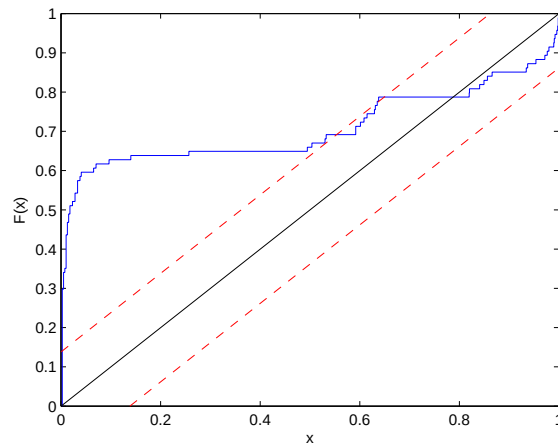
Kuva 2.44: Muunnettuihin odotusaikoihin perustuvan suureen U_k empirinen jakauma (sininen viiva) tasajakautumaa vastaan luottamusväleineen; u = 96 .
