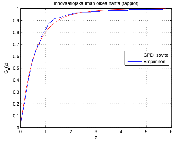
Kuva 4.7: Innovaatiojakauman oikea häntä, vastaten tappioita.
