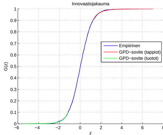
Kuva 4.6: Empiirinen innovaatiojakauma sovitetuilla GPD-hännillä.
