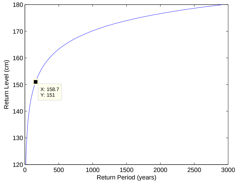
Kuva 2.9: Toistumistasokuvaaja vedenkorkeudelle GEV-mallissa.
