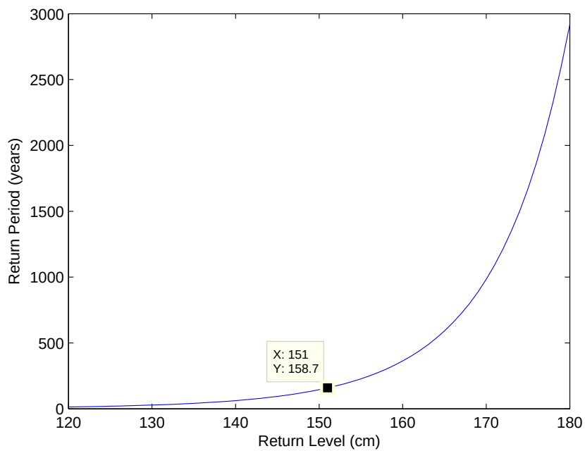
Kuva 2.10: Toistumisperiodokuvaaja vedenkorkeudelle GEV-mallissa.
