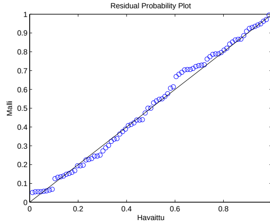
Kuva 2.54: Todennäköisyyskuvaaja mallille \mathcal{M}_1^N .
