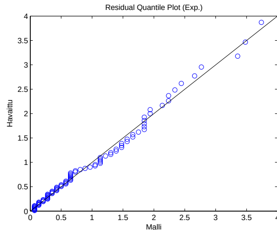
Kuva 2.41: Kvantiilikuvaaaja POT-mallille ( u = 96 ).
