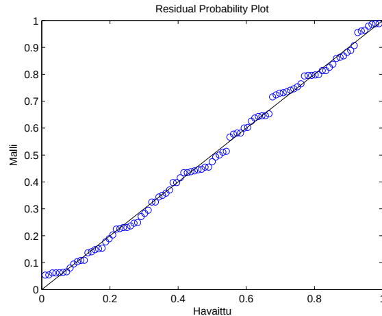
Kuva 2.50: Todennäköisyyskuvaaja mallille \mathcal{M}_2 .
