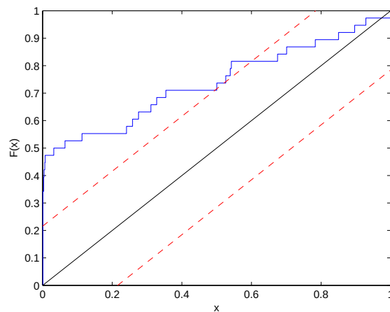
Kuva 2.45: Muunnettuihin odotusaikoihin perustuvan suureen U_k empirinen jakauma (sininen viiva) tasajakautumaa vastaan luottamusväleineen; u = 108 .
