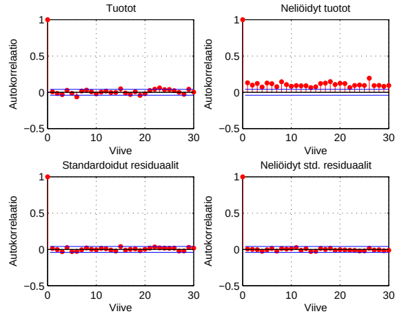
Kuva 4.3: Tuottojen ja neliöityjen tuottojen (ylärivi) sekä standardoitujen residuaalien ja näiden neliöiden (alarivi) autokorrelaatiofunktiot.
