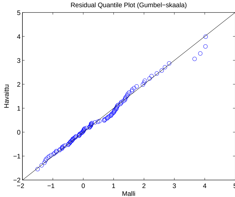
Kuva 2.38: Kvantiilikuvaaja trendin sisältävälle GEV-mallille.
