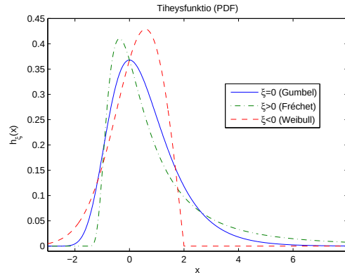
Kuva 1.1: GEV-jakauman tiheysfunktio.
