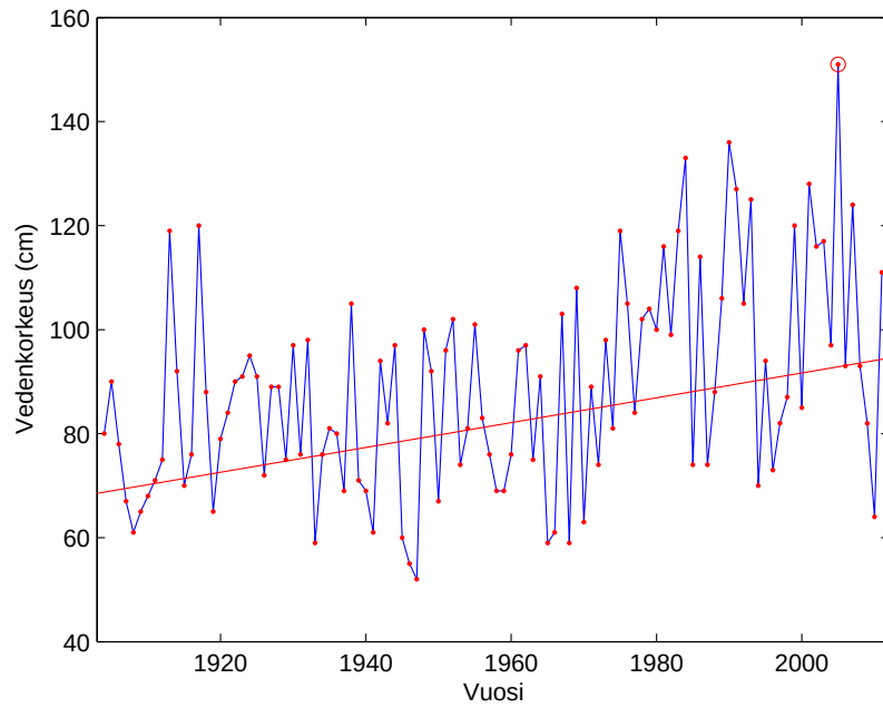
Kuva 2.36: Vedenkorkeuden vuosittaiset maksimit ja \mu(t) :n estimaatti.
