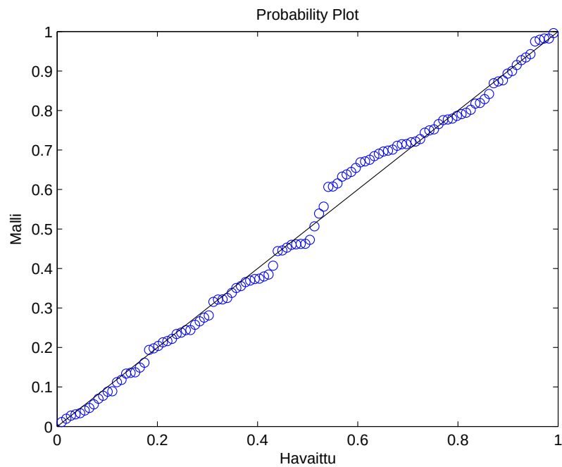
Kuva 2.37: Todennäköisyyskuvaaja trendin sisältävälle GEV-mallille.
