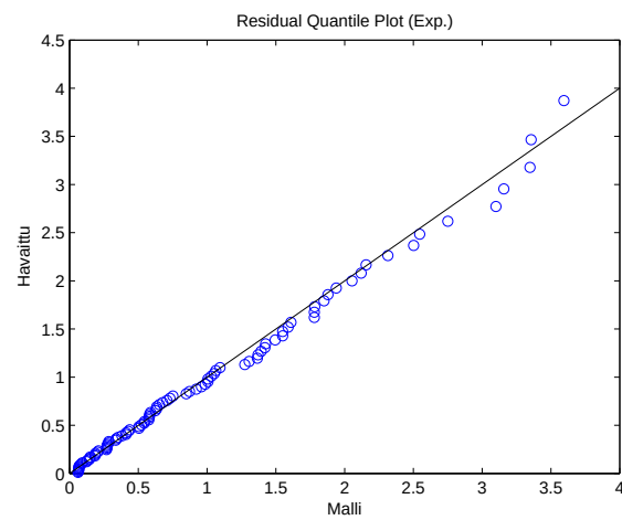
Kuva 2.49: Kvantiilikuvaaja mallille \mathcal{M}_1 .
