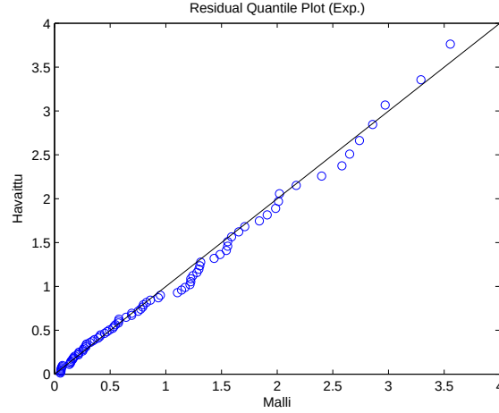
Kuva 2.55: Kvantiilikuvaaja mallille \mathcal{M}_1^N .
